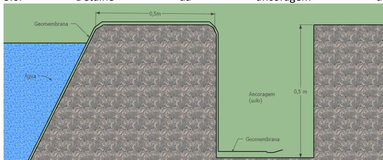
3.6. Detalhe da ancoragem das laterais da geomembrana.
